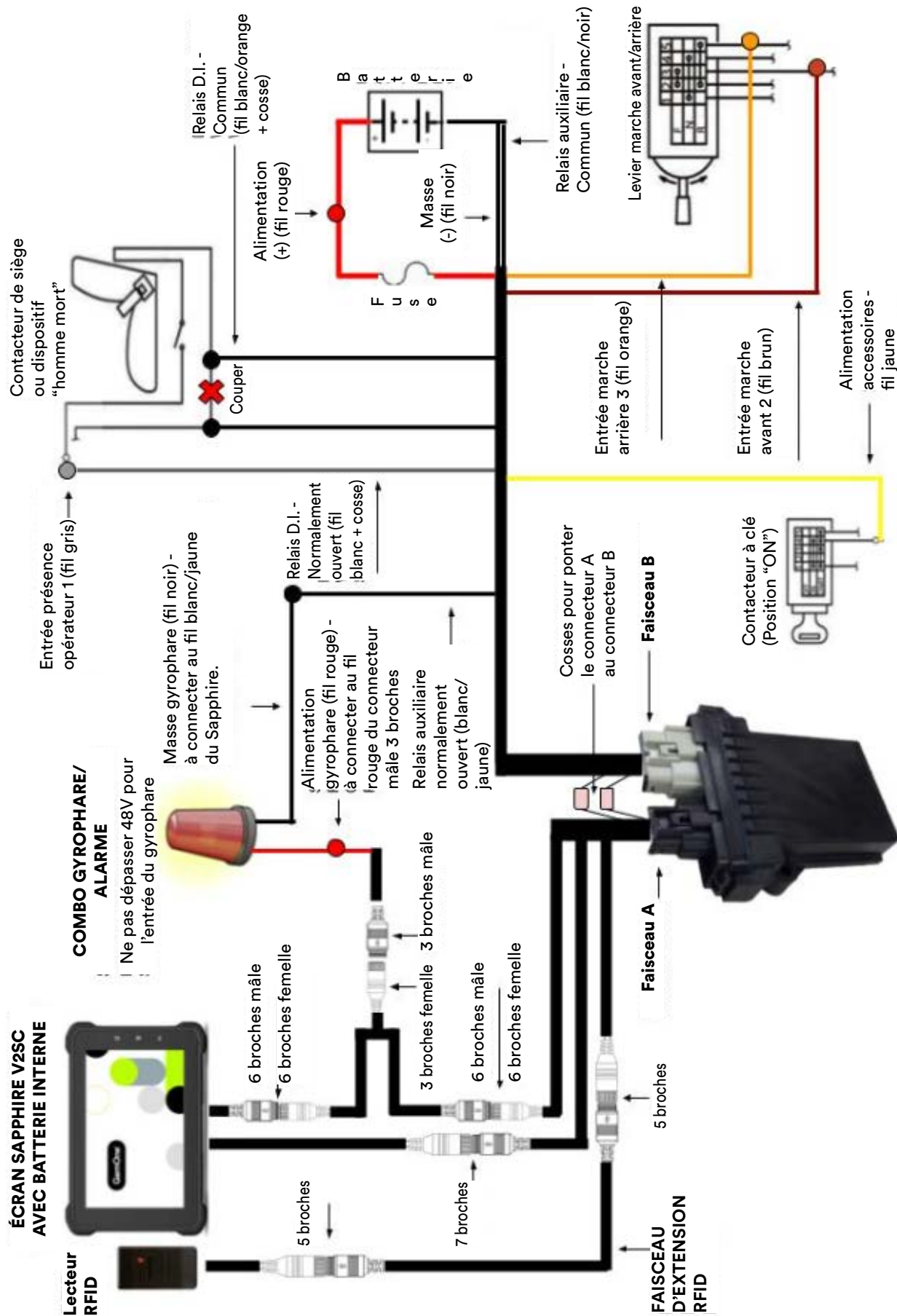
Schéma générique V2SC - 36-80V HV
